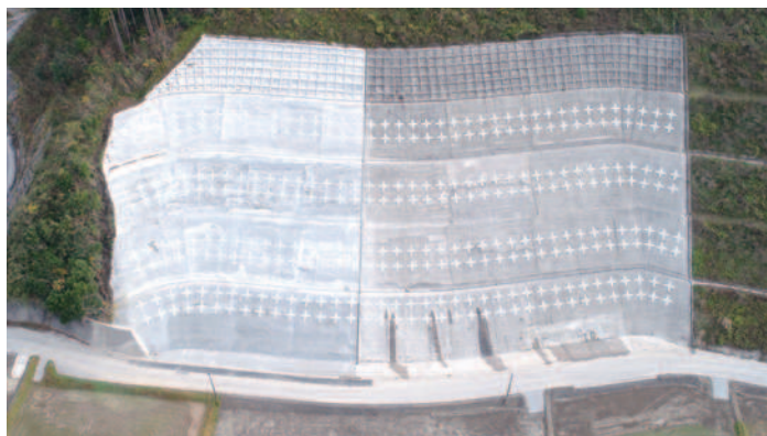
寺山法面保護工事 (宮崎県日南市)
